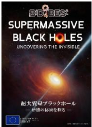
超大質量ブラックホール
