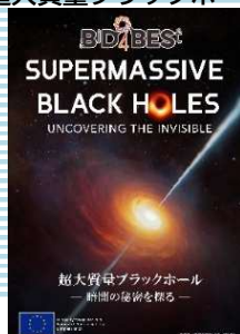
超大質量ブラックホール
